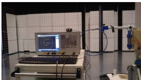
▲図3 E5061B/3L5 を使用した中・短波帯用自作ループアンテナ特性評価の様子
