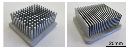
ヒートシンクの試作品
