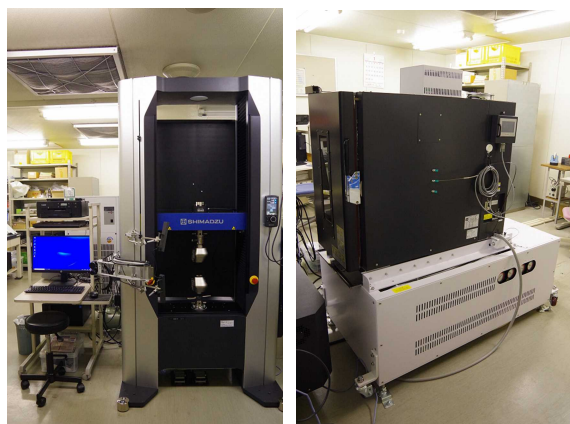
写真 導入機器事例（恒温槽付き精密万能試験機 伸び計付属（左）恒温槽（右）
