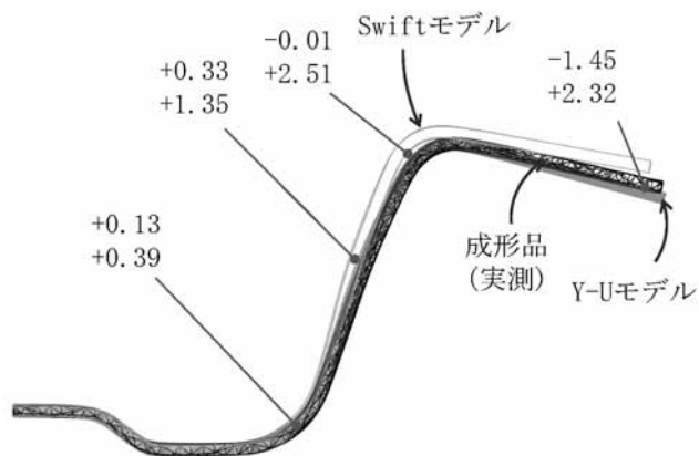
図2 ハット曲げ形状 数値は各箇所での実測との差 (mm) 上段：Y-Uモデル、下段：swiftモデル。
