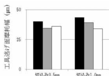
図8 工具摩耗量
