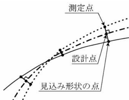
図3 見込み形状の点群データ作成
