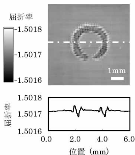
図8 レーザー加工部の屈折率分布推定
