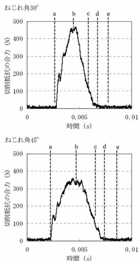
図3 切削抵抗
