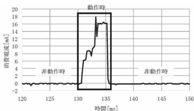
図1 データ送信時の消費電流
