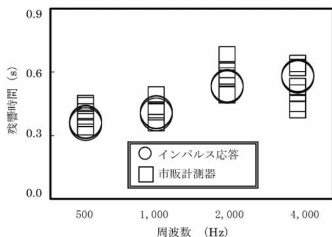
図3 残響時間計測結果の比較
