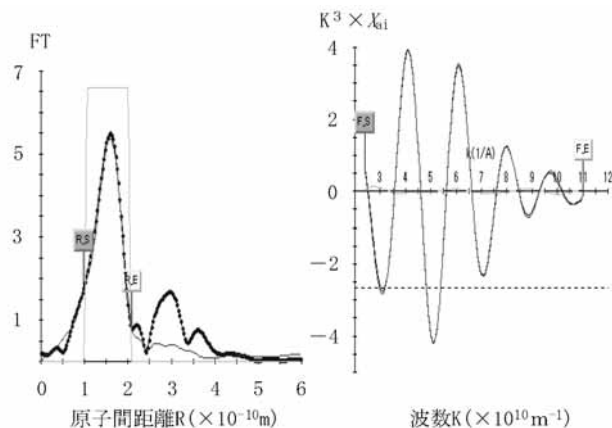
図4 めっき液②の硬X線XAFS測定 (EXAFSスペクトル) 左図の枠で囲った箇所の動径分布関数を逆フーリエ変換することで右図の特定シェルのEXAFS振動を抽出することができる。
