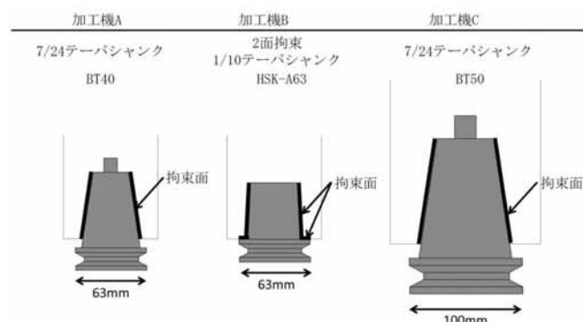
図2 加工機の工具シャンク形式
