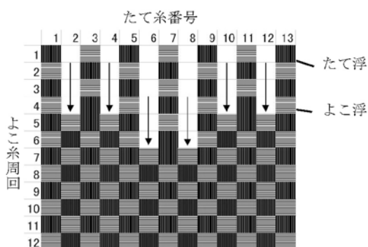
図2 たて糸挿入時の組織図 (平織)
