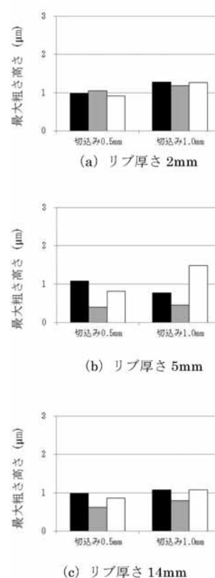
図14 リブ壁面の最大粗さ高さ（先端付近）
