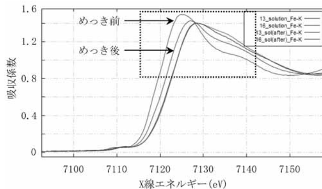
図13 めっき液④の硬X線XAFS測定 (XANESスペクトル)
