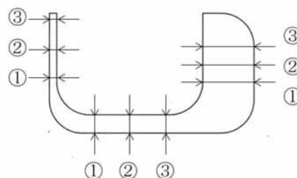
図3 リブ厚さ測定位置
