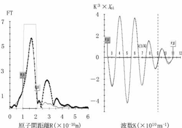
図5 めっき液③の硬X線XAFS測定 (EXAFSスペクトル) 左図の枠で囲った箇所の動径分布関数を逆フーリエ変換することで右図の特定シェルのEXAFS振動を抽出することができる。
