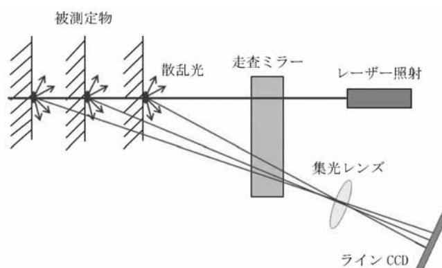
図 1 レーザーセンサの構造
