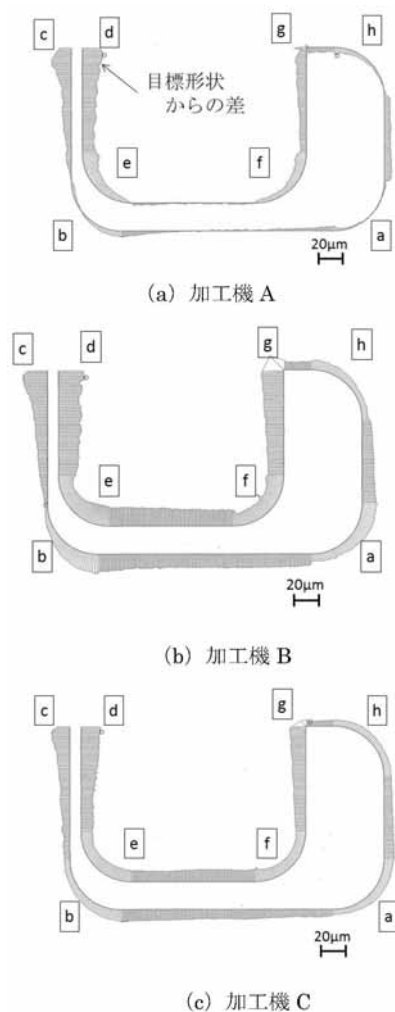
図12 工作物の輪郭プロファイル 測定位置：上面から1mm
