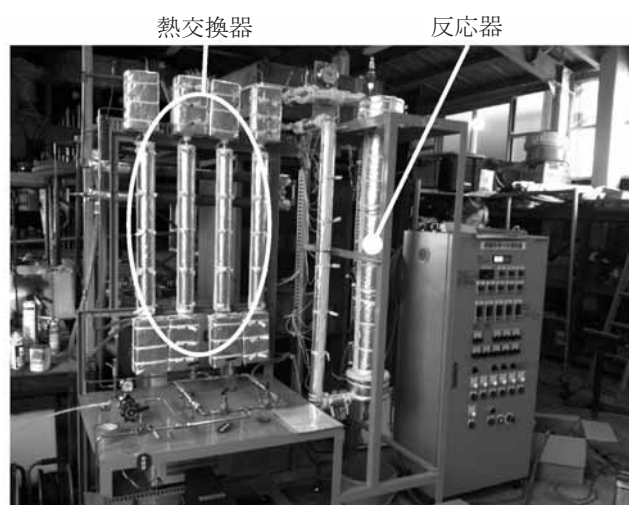
写真1 水熱処理装置（処理容量：3L）
