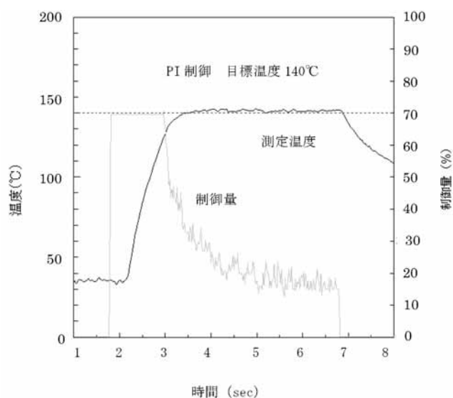
図2 パワー制御（設定温度と制御量）
