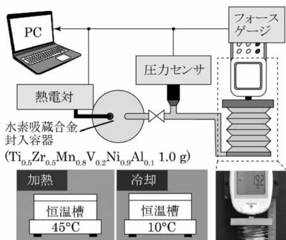
図1 アクチュエータの動作特性評価用セットアップ
