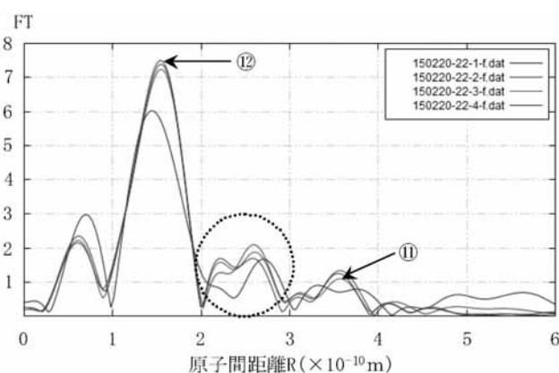
図12 硬X線XAFS測定 (EXAFSスペクトル)
